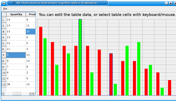
Figure 9.8. /examples/ModelView/TableView
